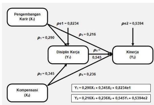
Gambar 6. Diagram Jalur Gabungan
