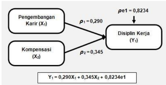
Gambar 2. Diagram Jalur Model Struktur II
