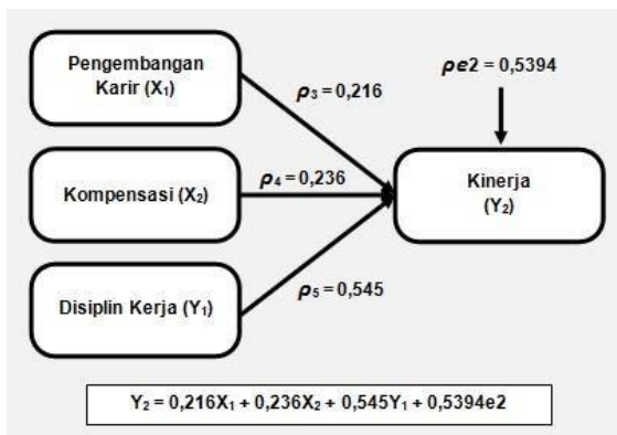
Gambar 3. Diagram Jalur Model Struktur II
